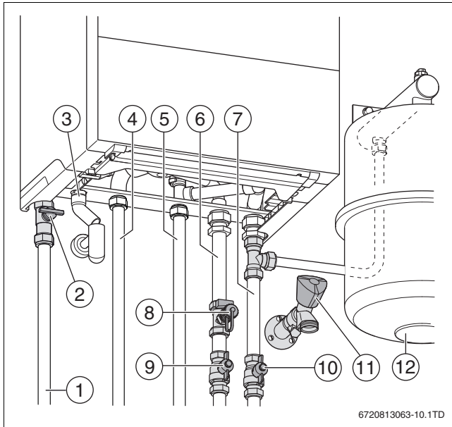
Bild 1 Anschlusszubehör (Beispiel)
